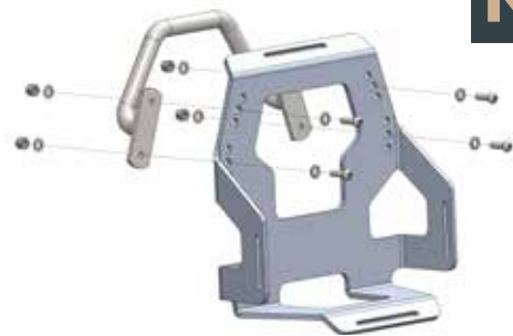
Montage am C-Bow Grundhalter
